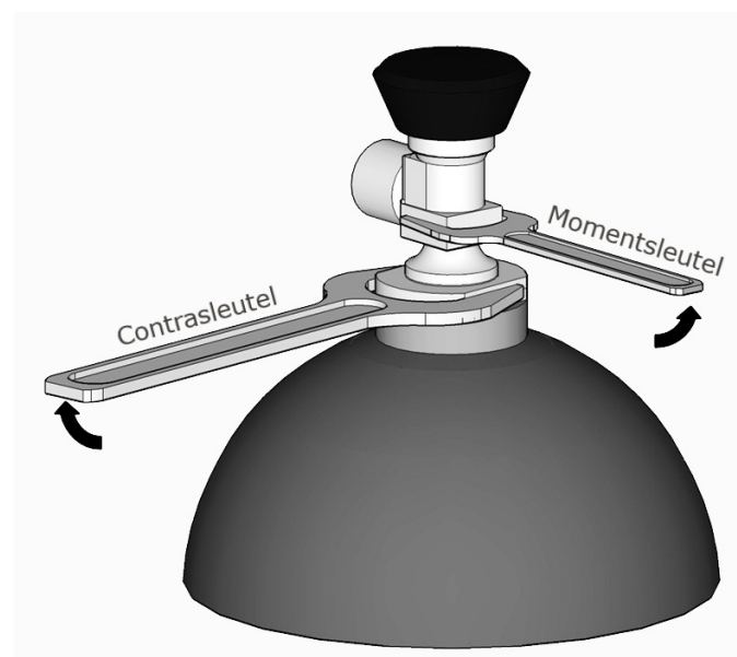
Afbeelding 3. Gebruik van de kontrasleutel om het ventiel te verwijderen
