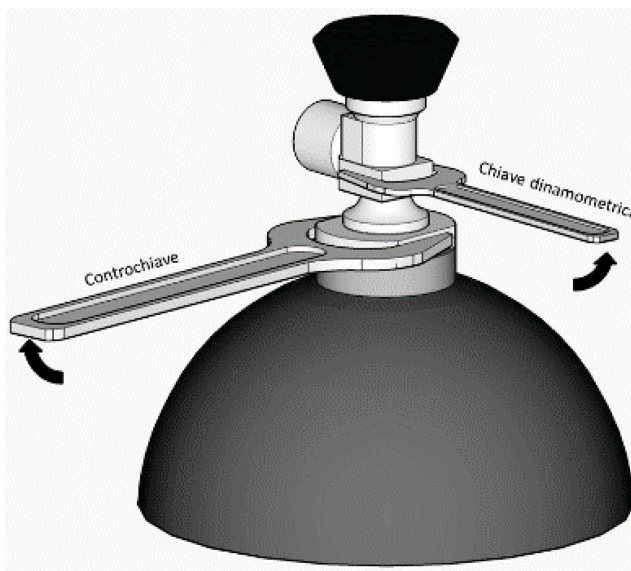
Slika 3. Ventil odstranite s pomočjo protiključa
