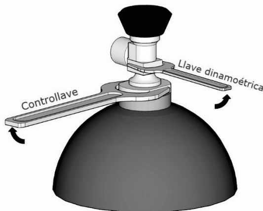
Figura 3. Uso de la contrallave para el desmontaje de la válvula.
